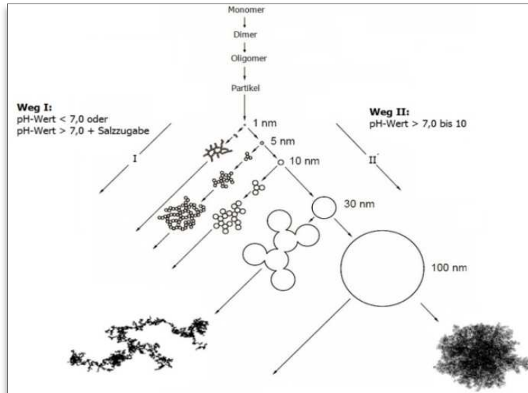
Abb.1: Kondensation der Kieselsäure in Anlehnung an [6]
