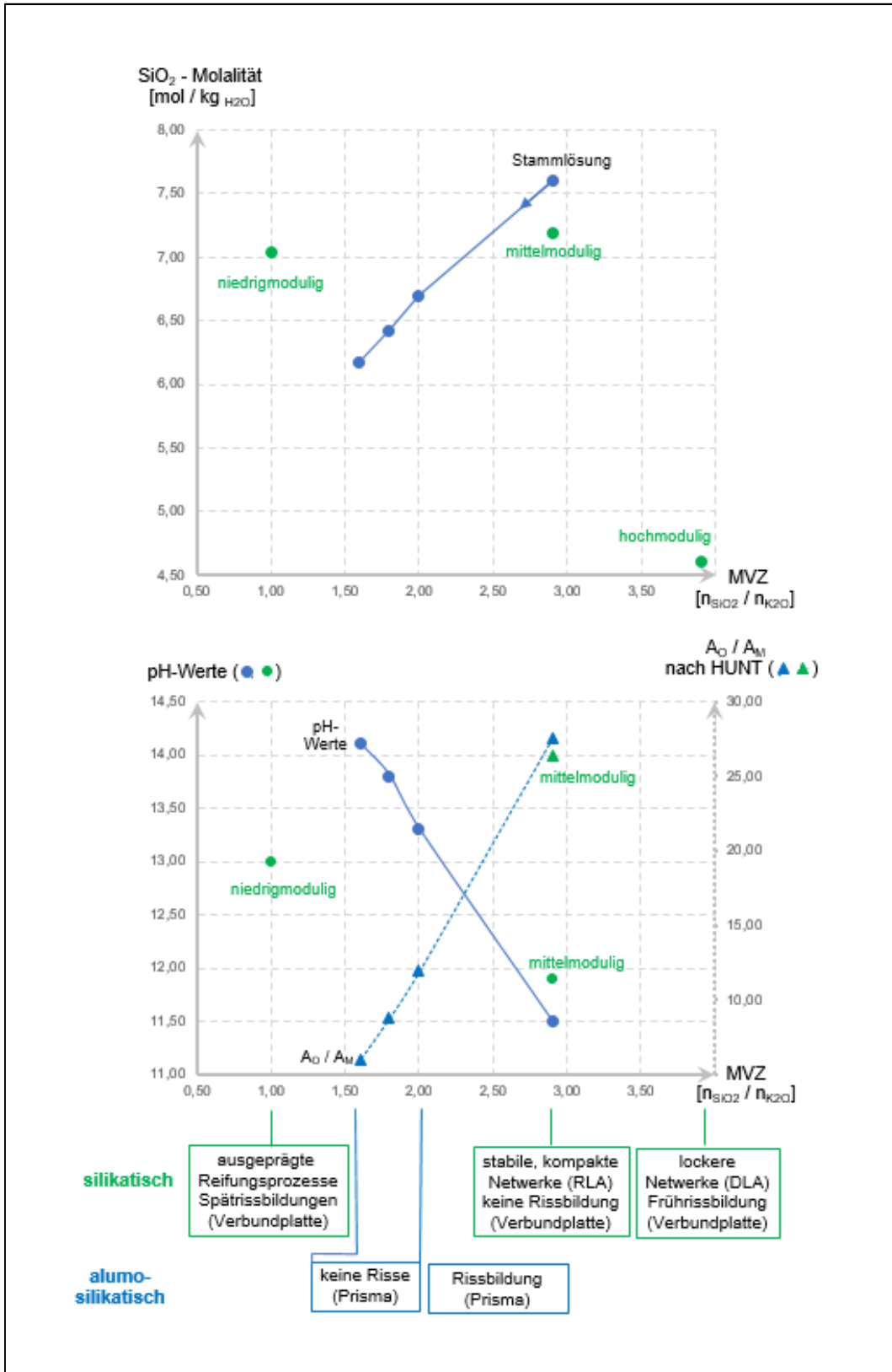
Abb. 3 : Kalium-Wasserglaslösungen in Abhängigkeit von MVZ und SiO 2 -Molalität (oben); MVZ, pH-Wert und A 0 /A M -Verhältnis (unten) für silikatische [2] und alumosilikatische [10] Binder
