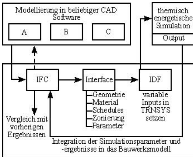
Bild 1. Workflow der entwickelten Schnittstelle von der Modellierung des Gebäudemodells über die Anreicherung mit bauphysikalischen Parametern zur thermisch-energetischen Simulation bis zur Rückführung und Einordnung der Simulationsergebnisse in das IFC-Modell
