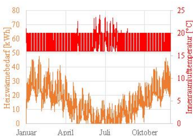
Bild 7. Ergebnis einer Jahres-Simulation des Testgebäudes, basierend auf stündlicher Auflösung Fig. 7. Result of an annual simulation for the test building, based on hourly resolution
