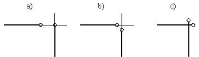
Bild 4. Modellierungsbedingte fehlerhafte Verschneidungen von Wandachsen, falls durch Abstände (a, b) oder Überlappungen (c) keine deckungsgleichen Endpunkte vorliegen, müssen automatisch korrigiert werden
