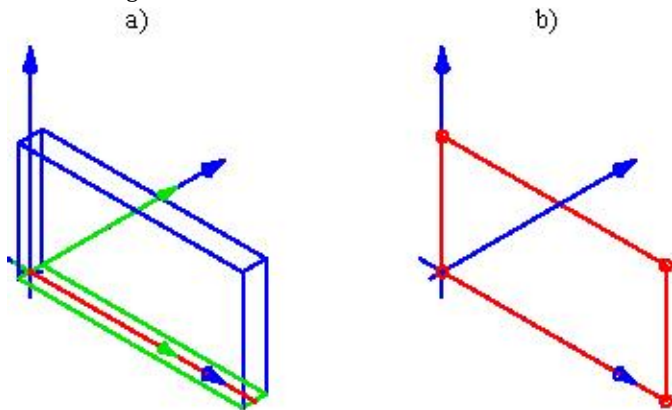
Bild 3. Definition der Wandgeometrien in IFC (a) aus Grundfläche der Extrusion (grün), Volumenkörper aus Extrusion (blau) und Wandachse (rot) verglichen mit der Form in IDF (b) aus vier Eckpunkten der Wandfläche im 3-dimensionalen Raum (rot)
