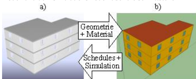
Bild 5. Visualisierung des fiktiven Testgebäudes als IFC im Viewer von APSTEX (a) und als konvertierte IDF in SketchUp (b)
